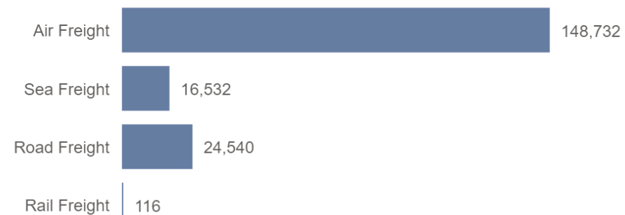
NO2 WTW (kg)
