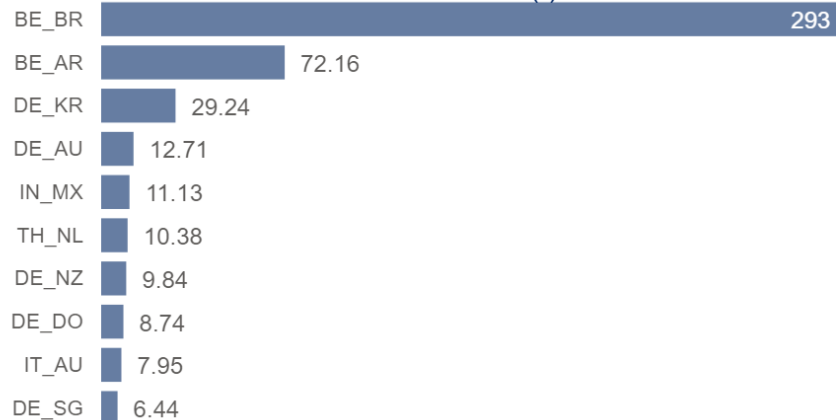
CO2e WTW (t)
