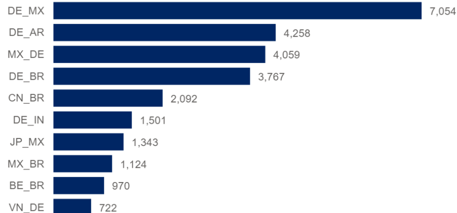
CO2e WTW (t)
