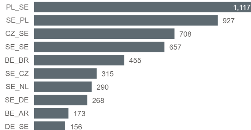
CO2e WTW (t)
